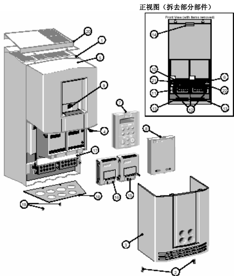
图 2—3 690+ 交流变频器，D规格 15 — 22KW
