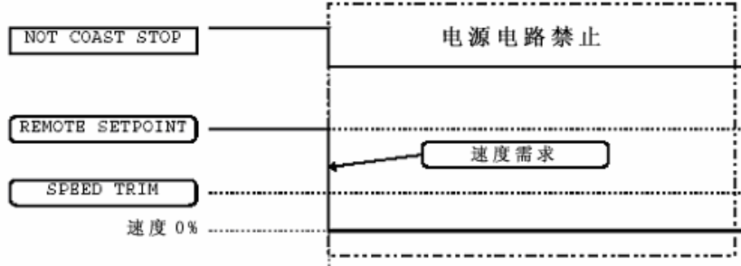
图 4—10 强制自由停止举例
