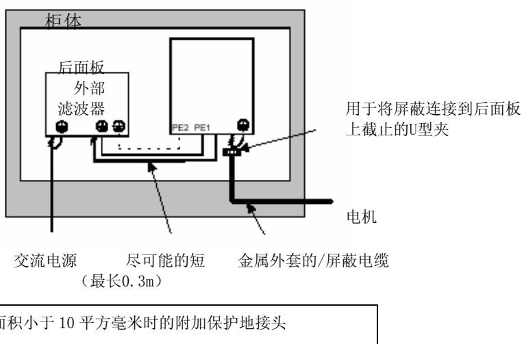
图 9-1 电磁兼容和安全接地电缆布线
