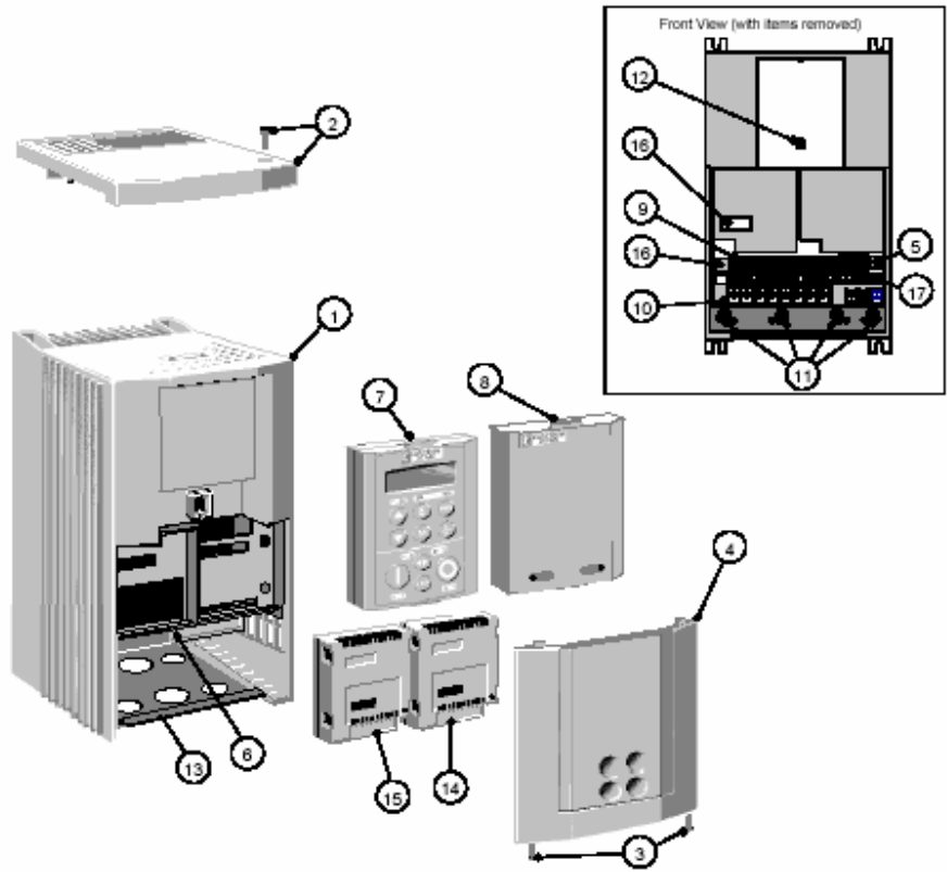
正视图（拆去部分部件）
