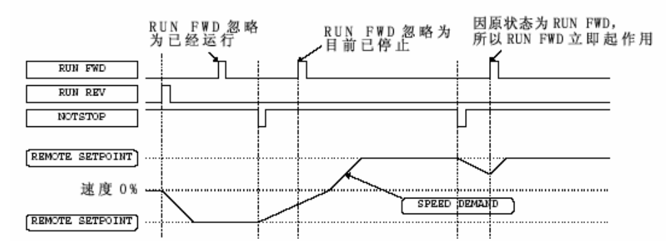
图 4—11 RUN FWD、RUN REV和NOT STOP参数之间的相互作用
