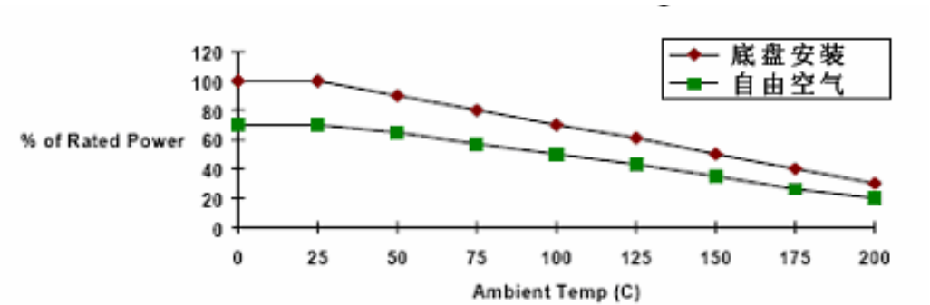
图 3—19 制动电阻额定值图表
