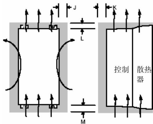
强制空气流
