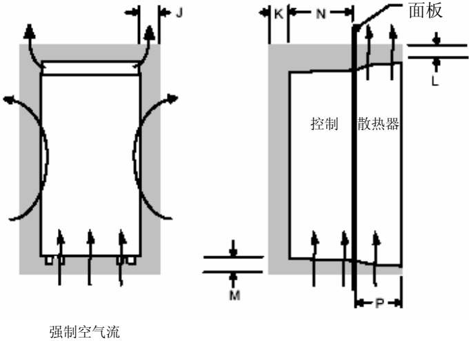
图 3—6 法兰板安装式产品/应用
