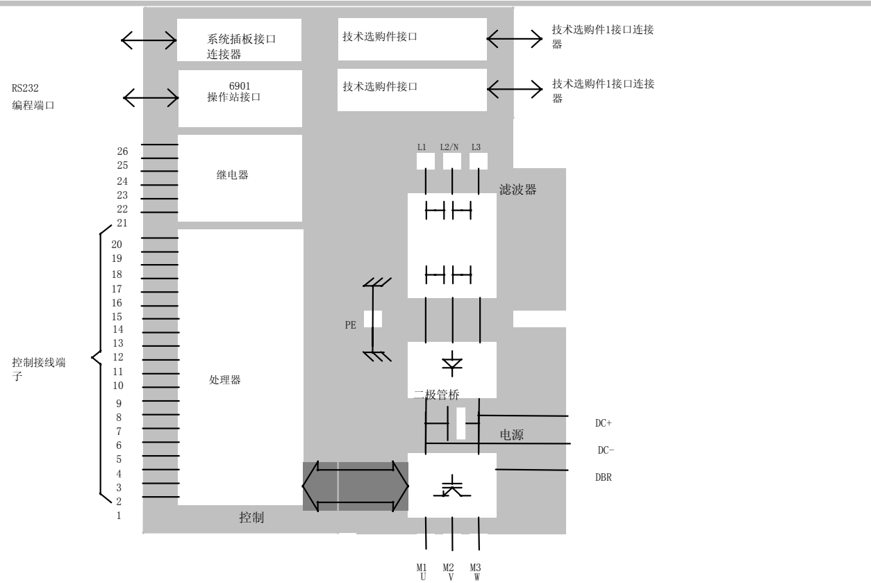
图2-6 功能框图(B规格)
