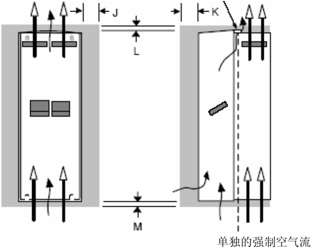
图 3—11 壁挂式产品/应用的空气间隙
