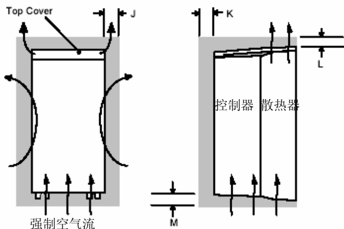
图 3—5 壁挂式产品/应用的空气间隙
