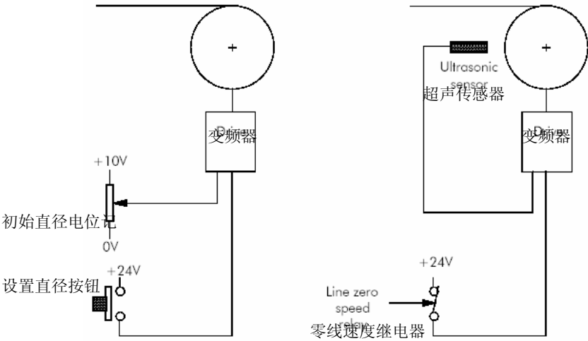
图 10—3 卷取直径
