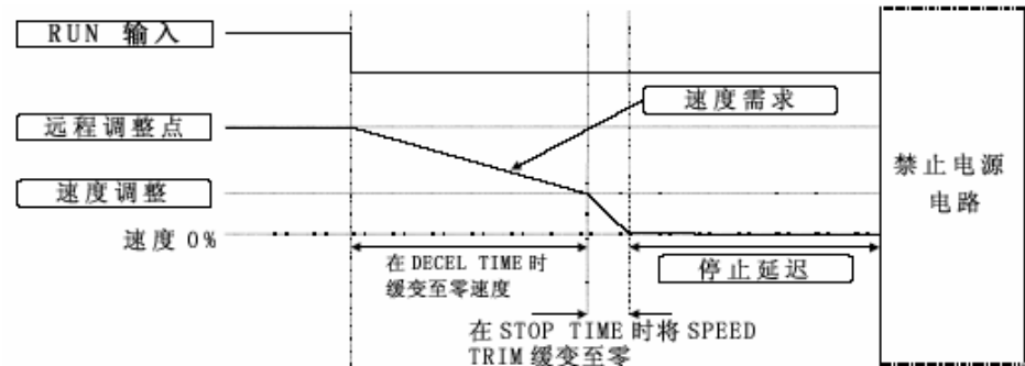
图 4—6 利用远程控制斜坡至停止状态
