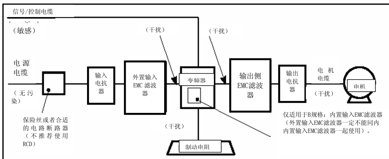
图 3-14 电缆布线要求
