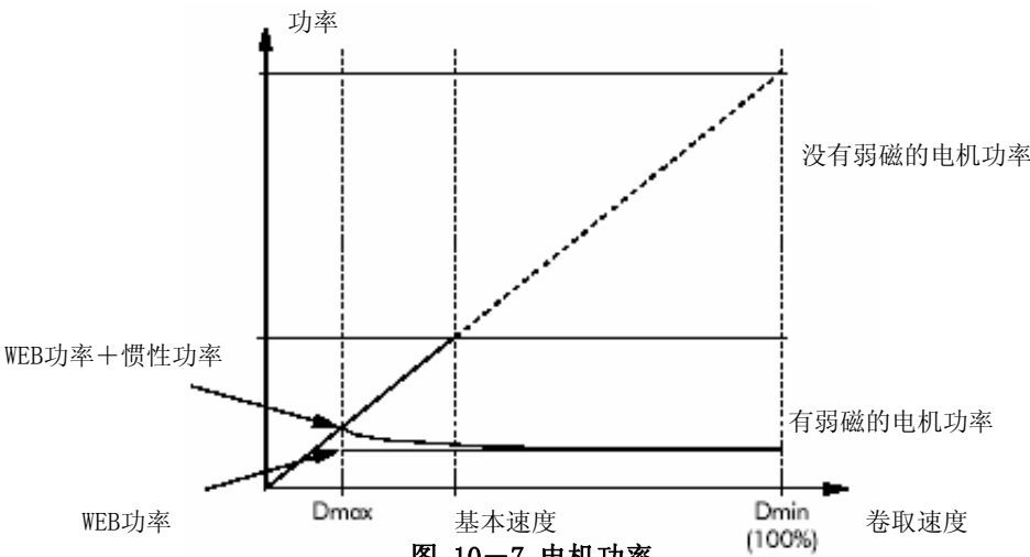
图 10-7 电机功率
