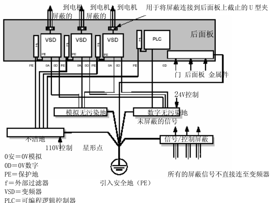
图 9-2 星形点接地
