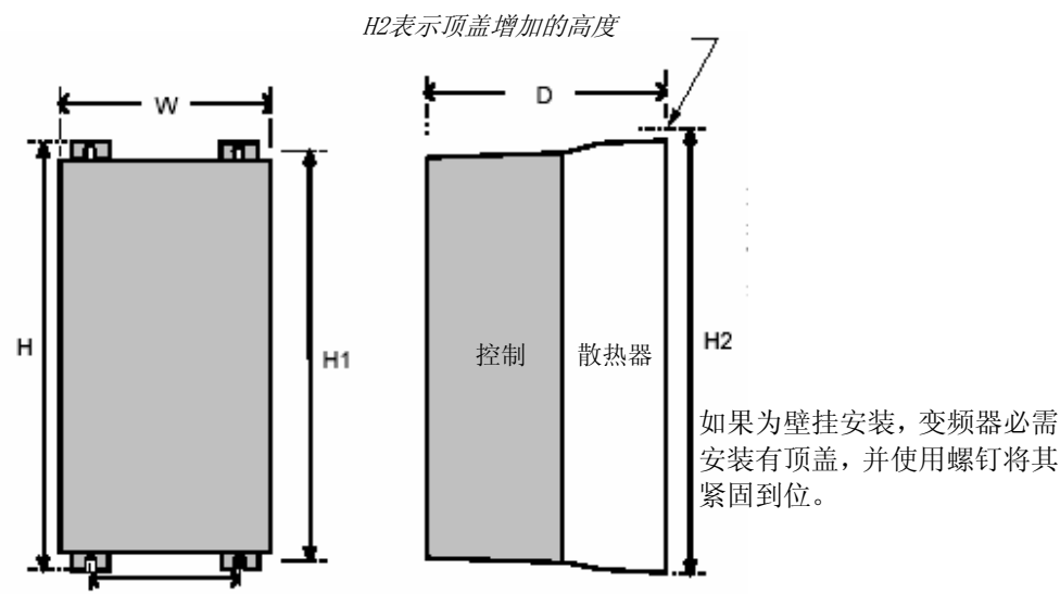
图 3—1 690+ 系列的机械尺寸
